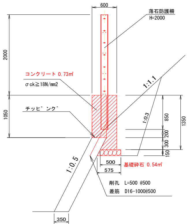
断面図
